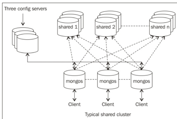
Figura 33. Sharding en un entorno de producción
