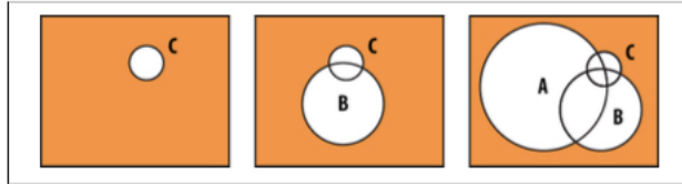
Figura 17. Restringiendo consultas OR de menor a mayor
