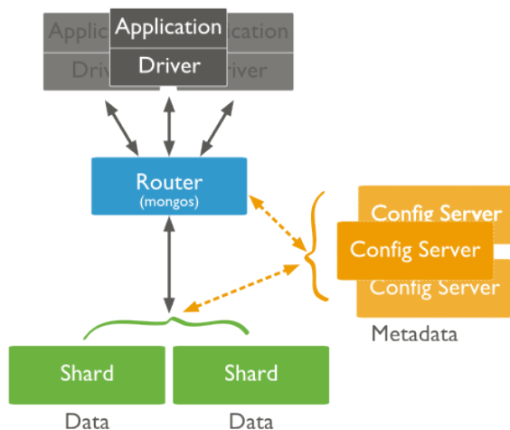
Figura 31. Componentes de un sharded cluster
