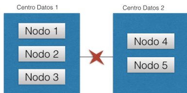
Figura 29. Elección de un nuevo primario
