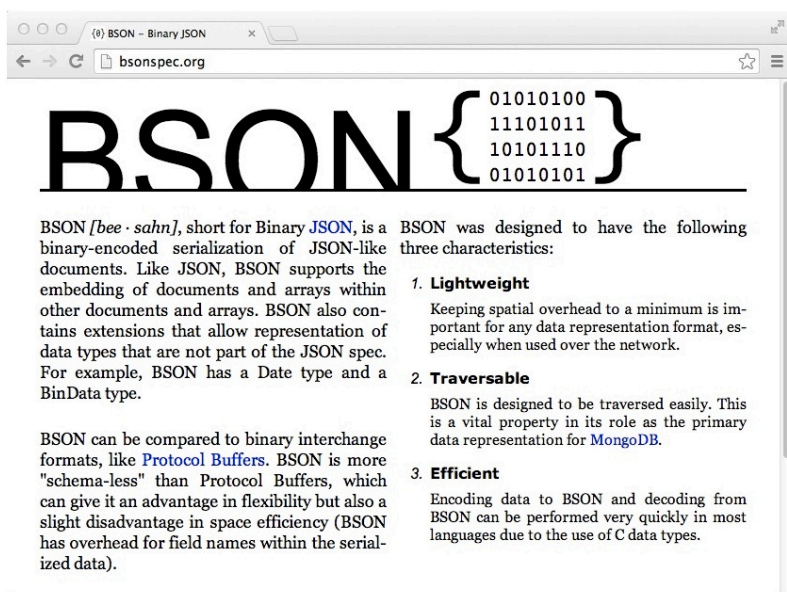
Figura 13. Especificación BSON
