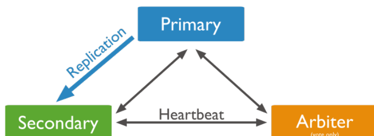
Figura 27. Arbitraje de un secundario
