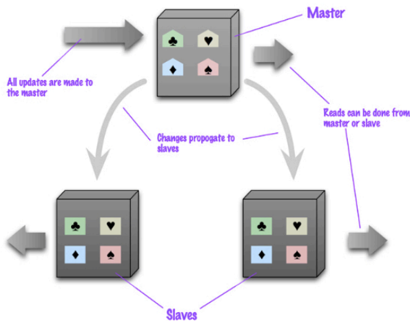
Figura 3. Replicación
