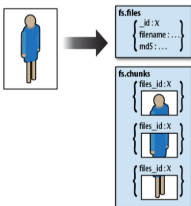
Figura 21. GridFS
