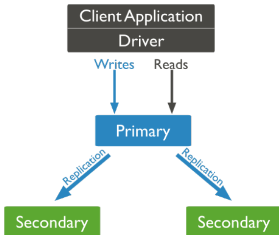
Figura 26. Conjunto de Réplicas
