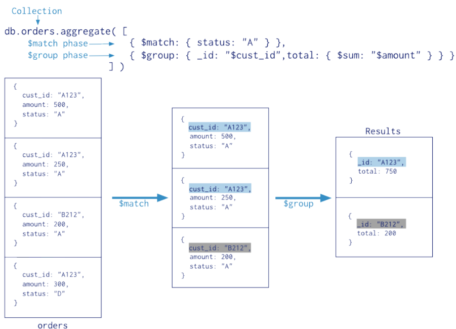
Figura 25. Ejemplo de pipeline con $match y $group
