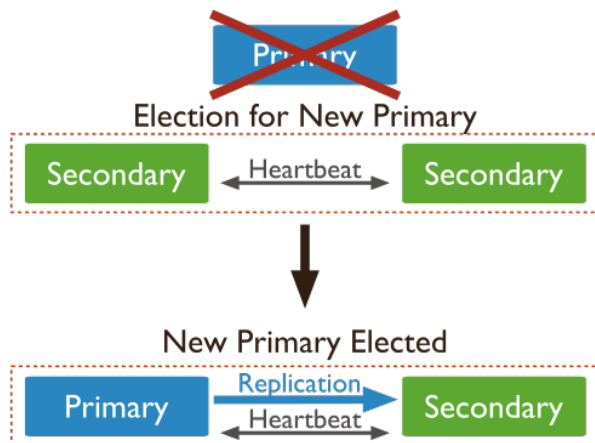
Figura 28. Elección de un nuevo primario
